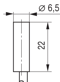
Габаритный чертеж
